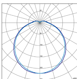
LUNA-430-IP65-25W
