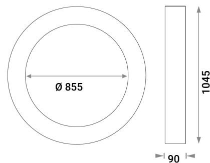
PLANET/N CIRCULAR ABIERTO 1045
