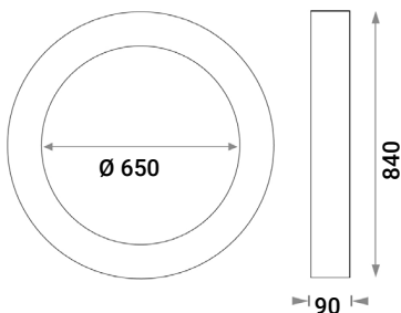
PLANET/N CIRCULAR ABIERTO 840
